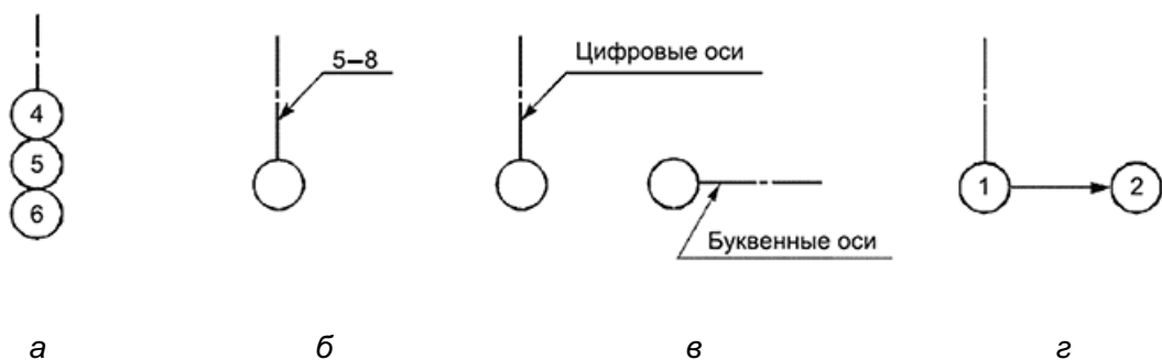
Рисунок 3 - Примеры ориентации координационной оси, к которой привязан элемент, по отношению к соседней оси
