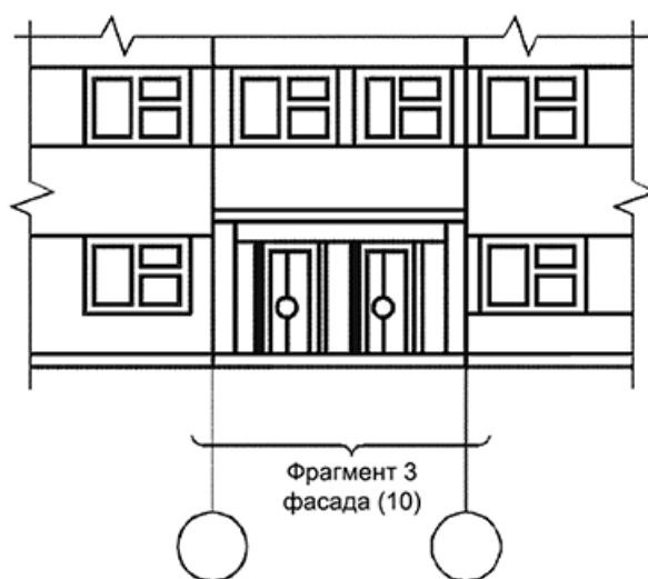
Рисунок 16 - Пример указания места размещения вынесенного фрагмента фасада
