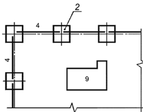
Рисунок 10 - Примеры нанесения номеров позиций или марок элементов
