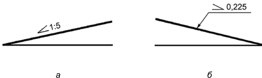
Рисунок 9 - Примеры обозначения уклона
