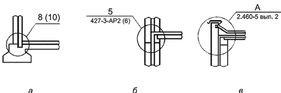
Рисунок 13 - Примеры указания мест расположения узла на плане, фасаде или разрезе
