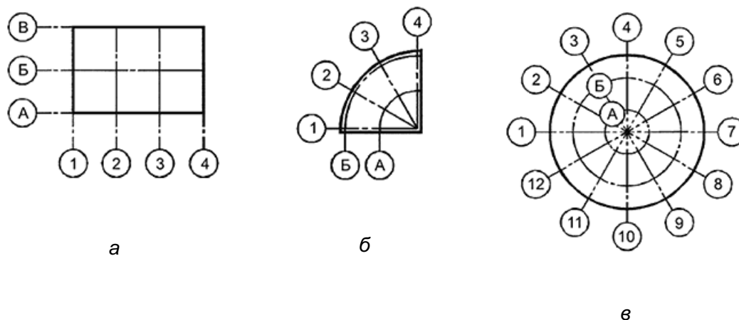
Рисунок 1 - Примеры обозначений координационных осей
