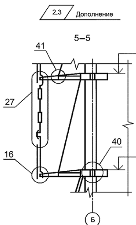
Рисунок Л.5 - Пример обозначения дополнительного изображения
