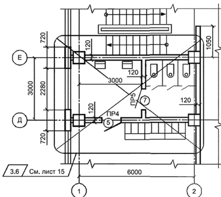
Рисунок Л.1 - Пример обозначения изменения части изображения
