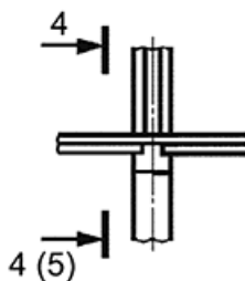
Рисунок 12 - Пример указания на чертеже секущей плоскости сечения
