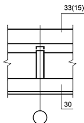
Рисунок 15 - Примеры размещения выносок по сечению конструктивных элементов
