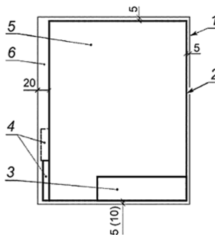
г) Для формата больше А4 при расположении надписи по короткой стороне листа
